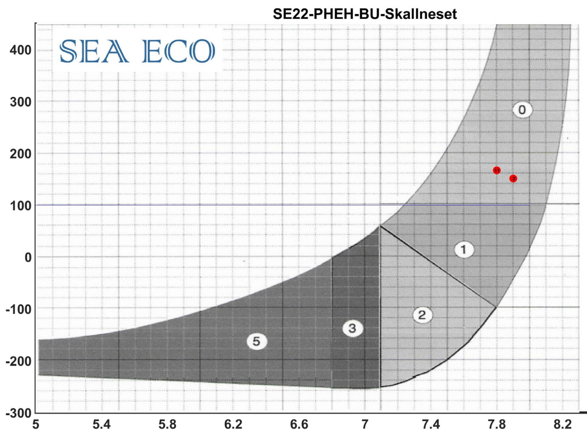
Figur 9 Forholdet mellom pH og E_h – målinger på lokaliteten beregnet med internutviklet programvare -bakgrunn er Figur D1:NS 9410.
